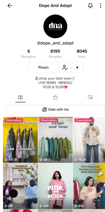
Gambar 4. Fitur TikTok.
